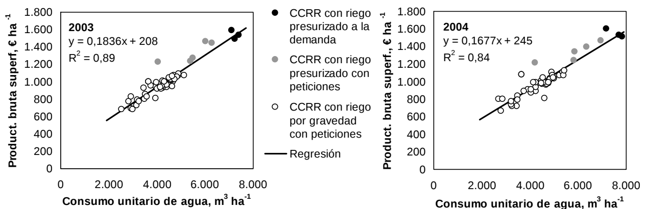
Figura 1. Relación entre el consumo unitario de agua y la productividad bruta por unidad de superficie por comunidades de regantes, según su tecnología de riego, durante las campañas 2003 y 2004 en Riegos del Alto Aragón.
